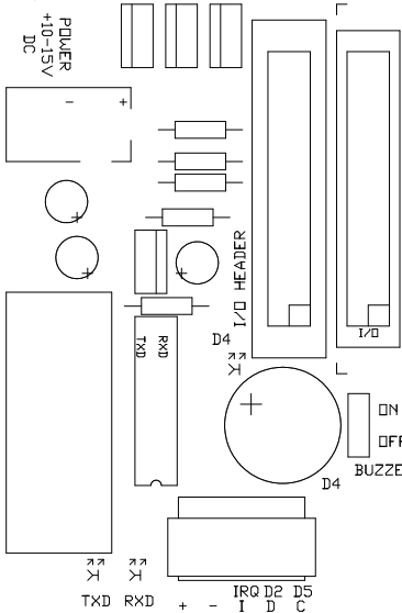
EVB_3A4 Top Overlay
